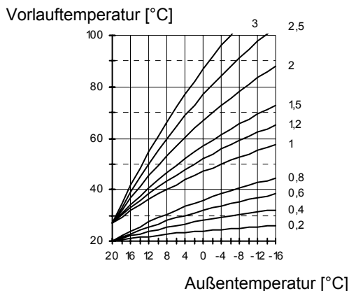
Heizkurvendiagramm (Einstellhilfe)
